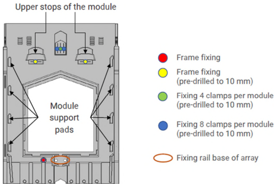
Figuur 2 – Frame, in diverse maten leverbaar
