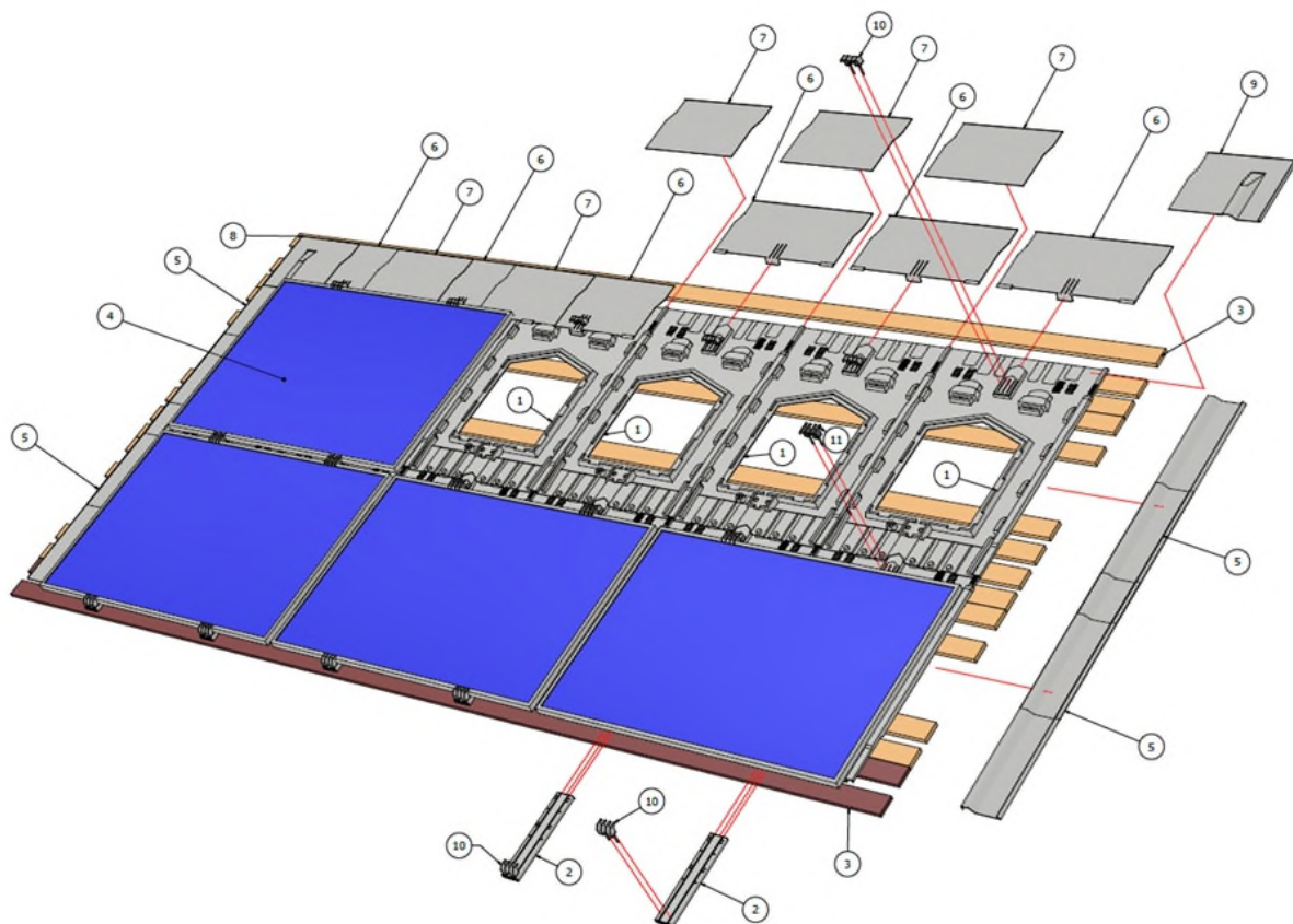
Figuur 1 – Systeemopbouw (één 'liggend' PV-paneel bedekt twee half-frames)
