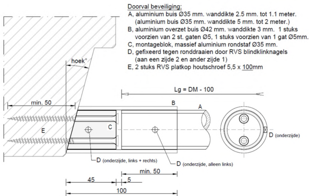
Figuur 2 – Doorvalbeveiliging, optie 2a/2b
